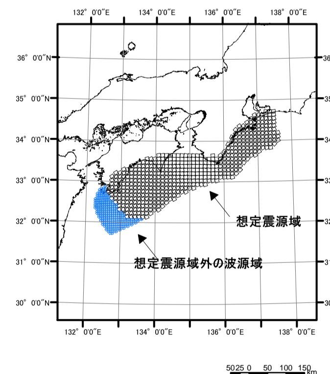
想定震源域と波源域の位置
