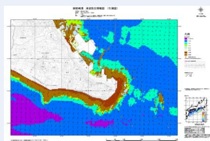
引潮図
